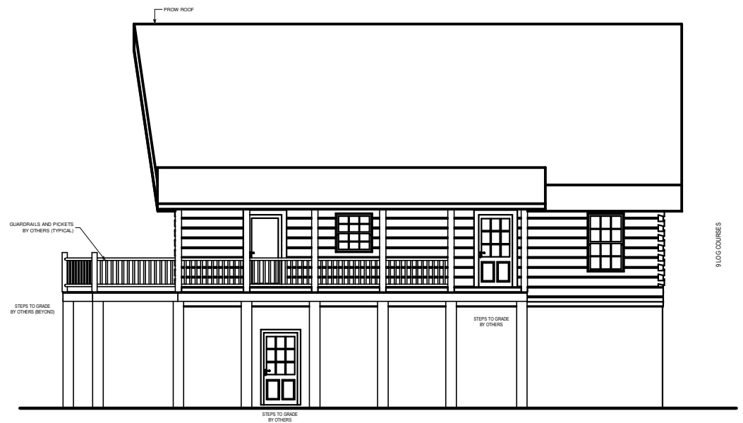
RIGHT ELEVATION
