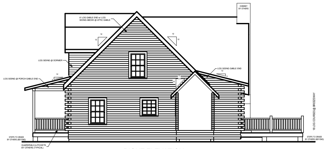
RIGHT ELEVATION
