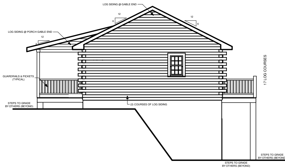
RIGHT ELEVATION
